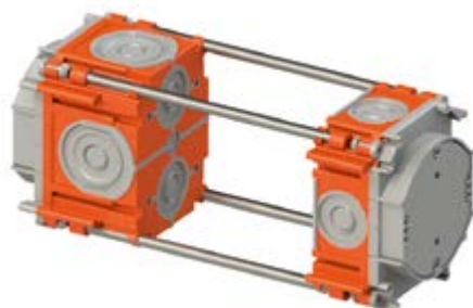
délka rozpěrných tyčí = tloušťka realizované stěny - 70 mm
