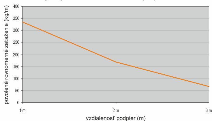
Graf znázorňuje maximálne povolené rovnomerné zaťaženie kábovej lávky v závislosti na vzdialenosti podpier
